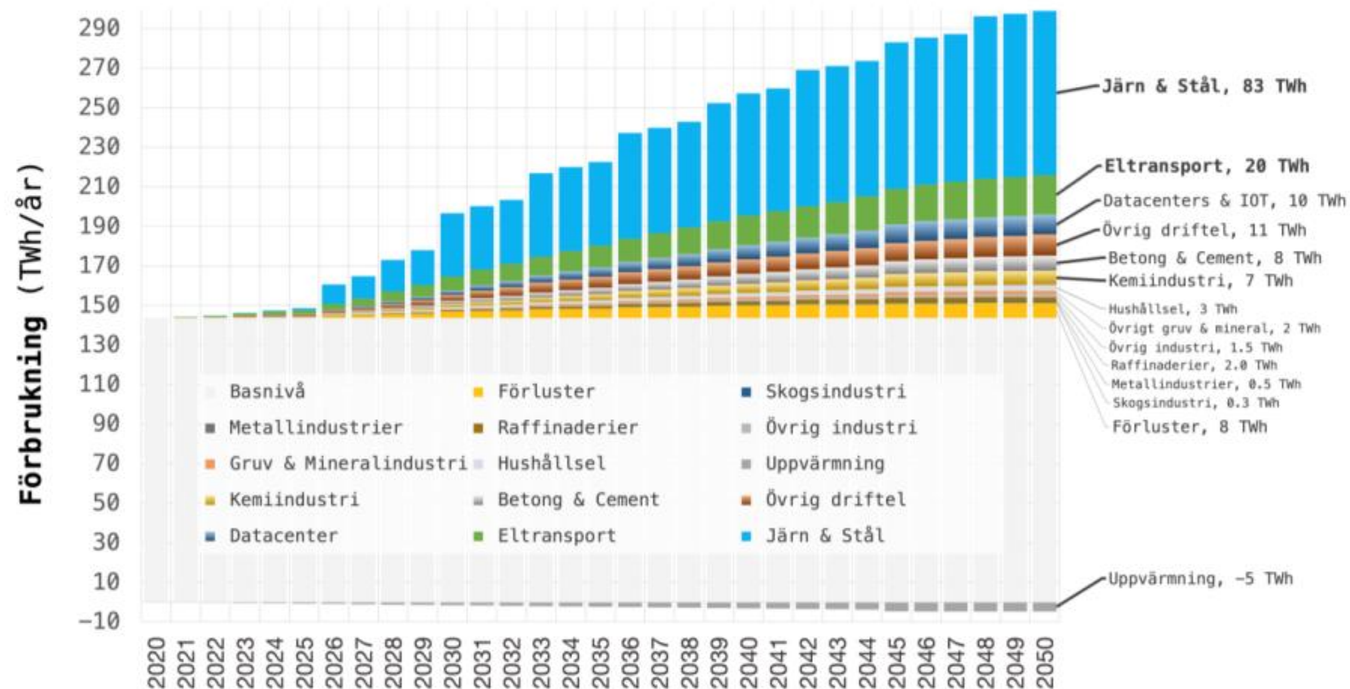
Figur 4, Referensscenario för förändrad elanvändning 2020 till 2050
